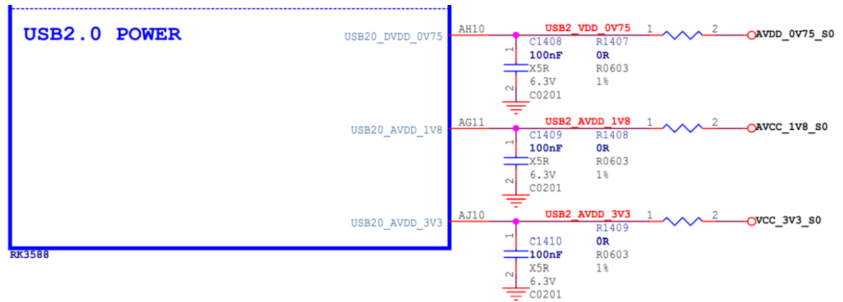
图 13 USB 2.0 PHY 供电电源
