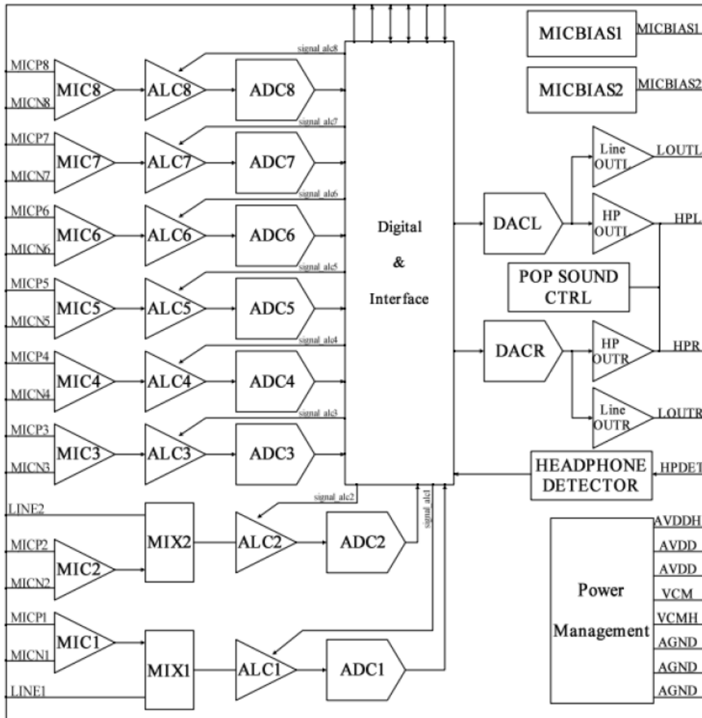
图 3-2 RK3308 codec
