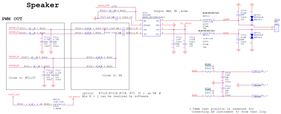
图 2-2 DSM PWM OUT 参考图
