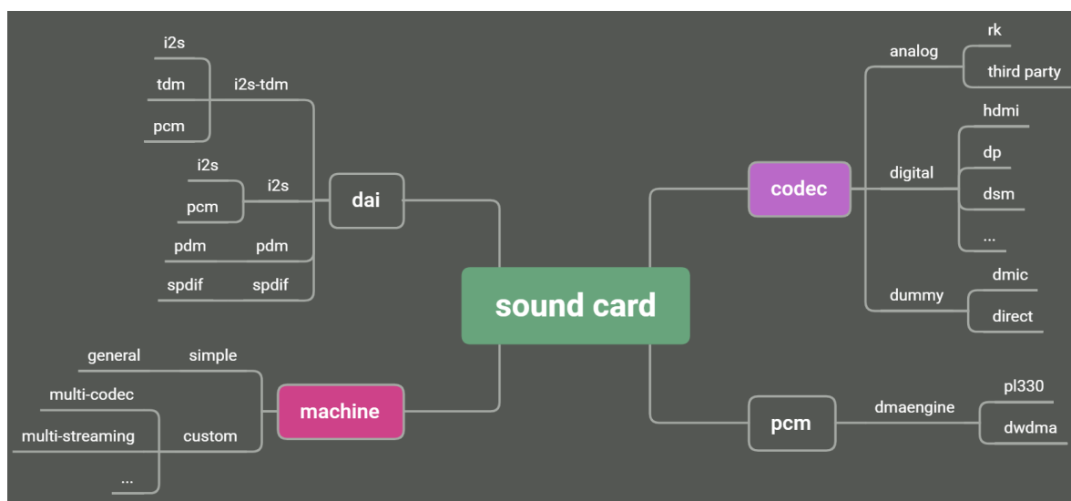
图 2-1 ALSA 声卡构成
