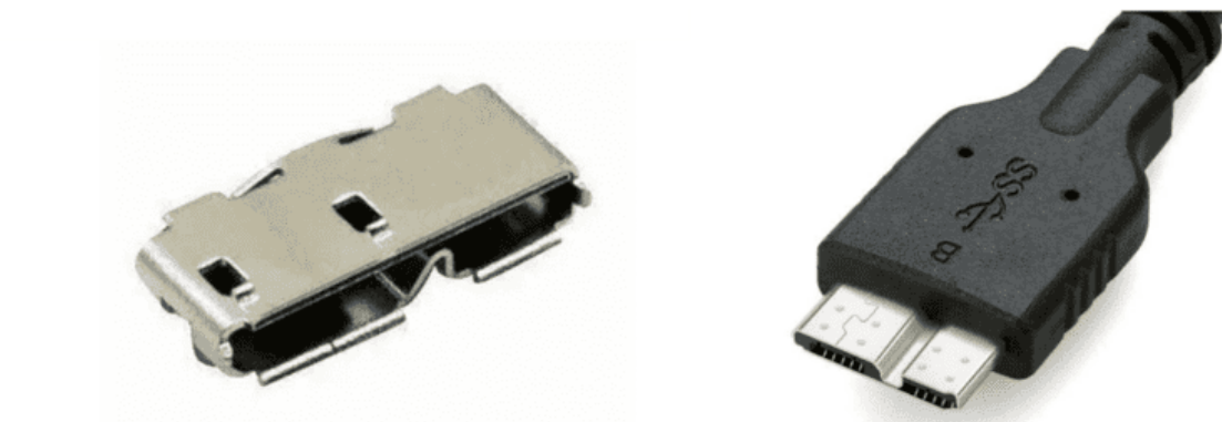
图 2-7 Micro USB 3.1 接口
