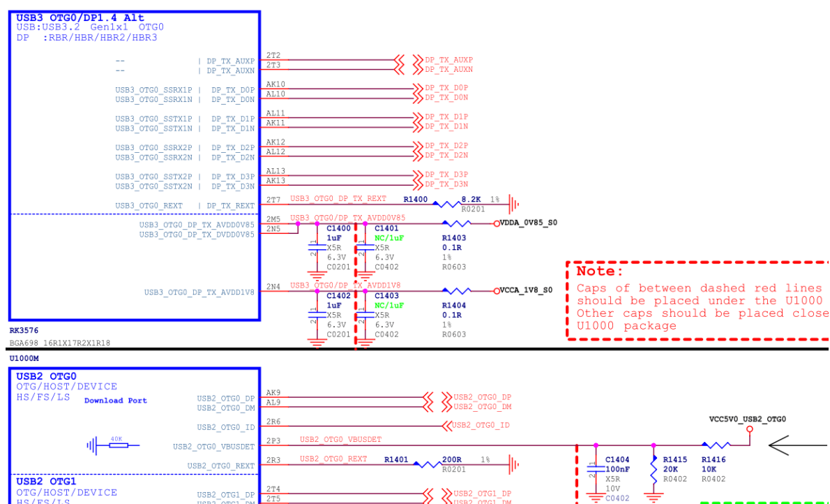
图 13 RK3576 Type-A USB 2.0/DP 电路
