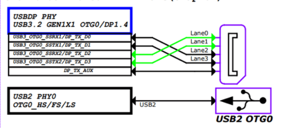
图 3 RK3576 OTG0 USB DP Path Map
