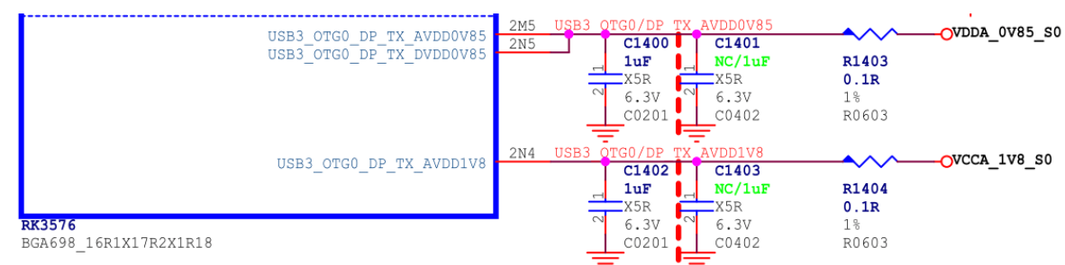
图 6 RK3576 USBDP Combo PHY 供电电源
