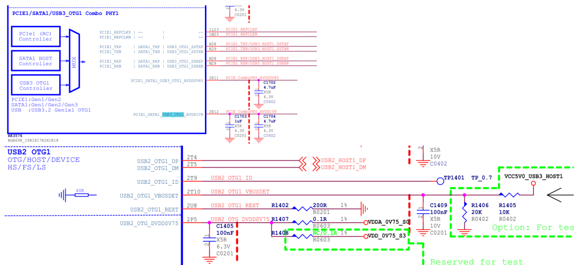
图 15 RK3576 USB3.1 OTG1 接口
